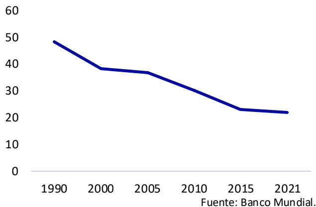
Figura 2: Coeficiente Gini
